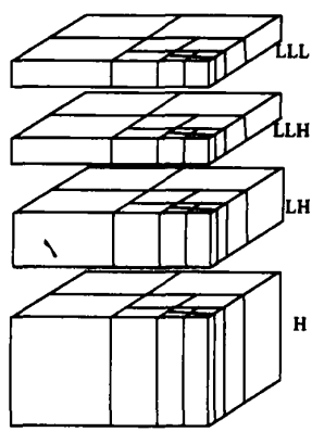
图3 最初楔形块结构
